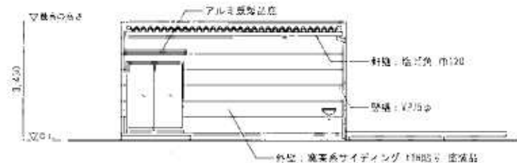
立面図 1/100
