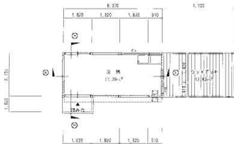
1 階平面図 1/100
