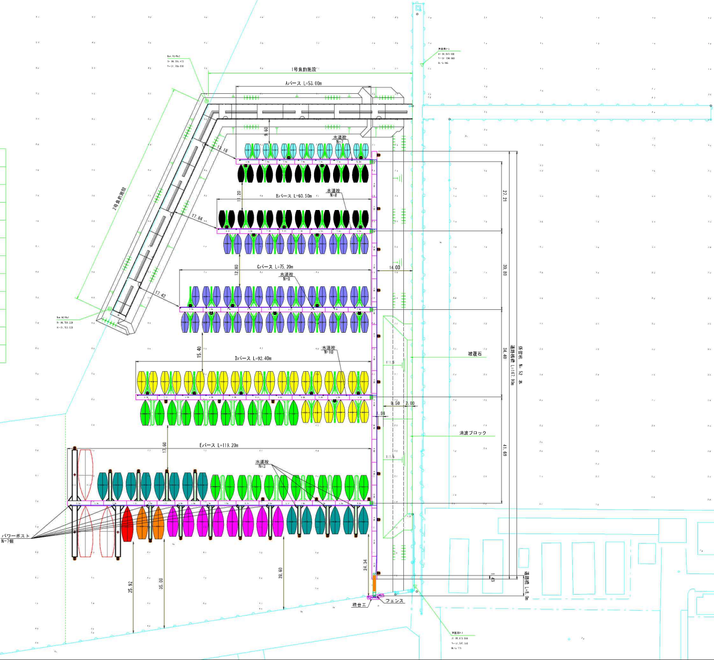
平面図
