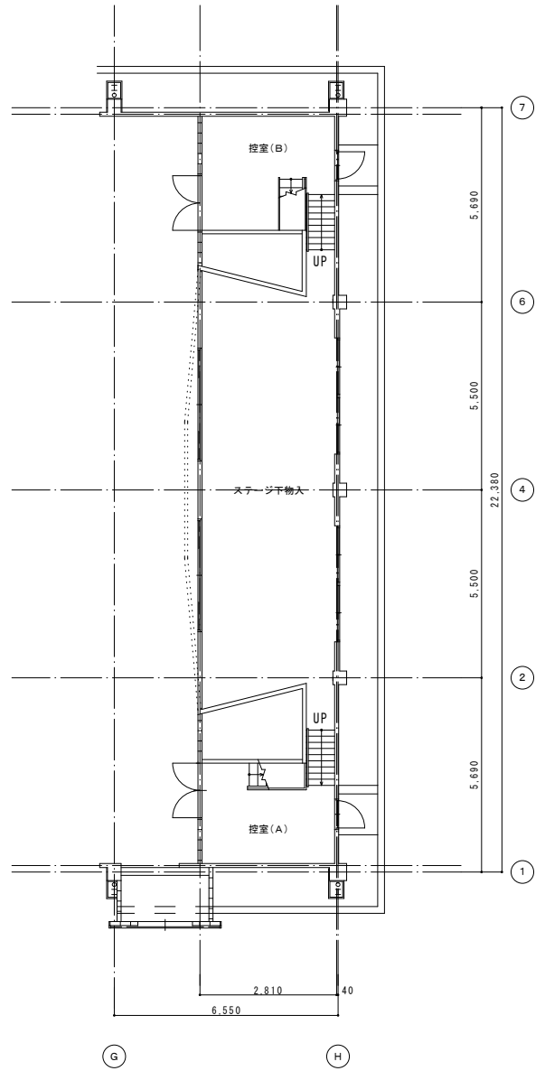
B 1階平面図 S=1/100
